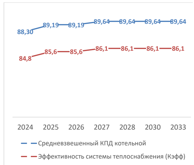
Рисунок 4 Прогнозируемая динамика усреднённого КПД котельных и эффективности СЦТ.
